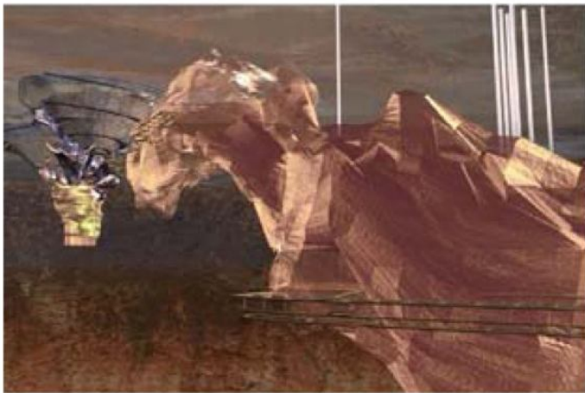
矿体模型和开拓系统
